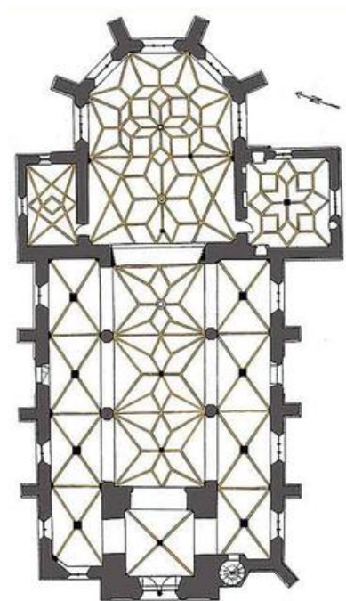
Grundriss und Deckenplan
